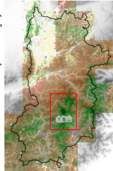
図1. 奈良県における大峯山と主な調査地(赤枠)。緑色は自然植生または代償植生、茶色は植林地、黄色は耕作地を示す(環境省による自然環境保全基礎調査より描く)。
